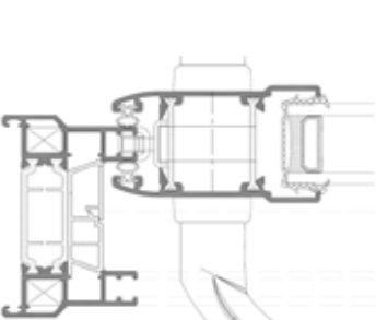
Jamb Detail
