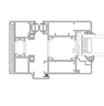
Jamb Detail
